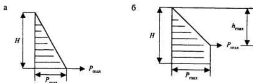
Рисунок Г.1 – Расчетные эпюры бокового давления бетонной смеси a – гидростатическое давление; b – расчетное давление при уплотнении смеси внутренними вибраторами
